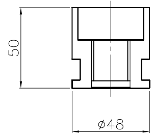
埋設用脚
